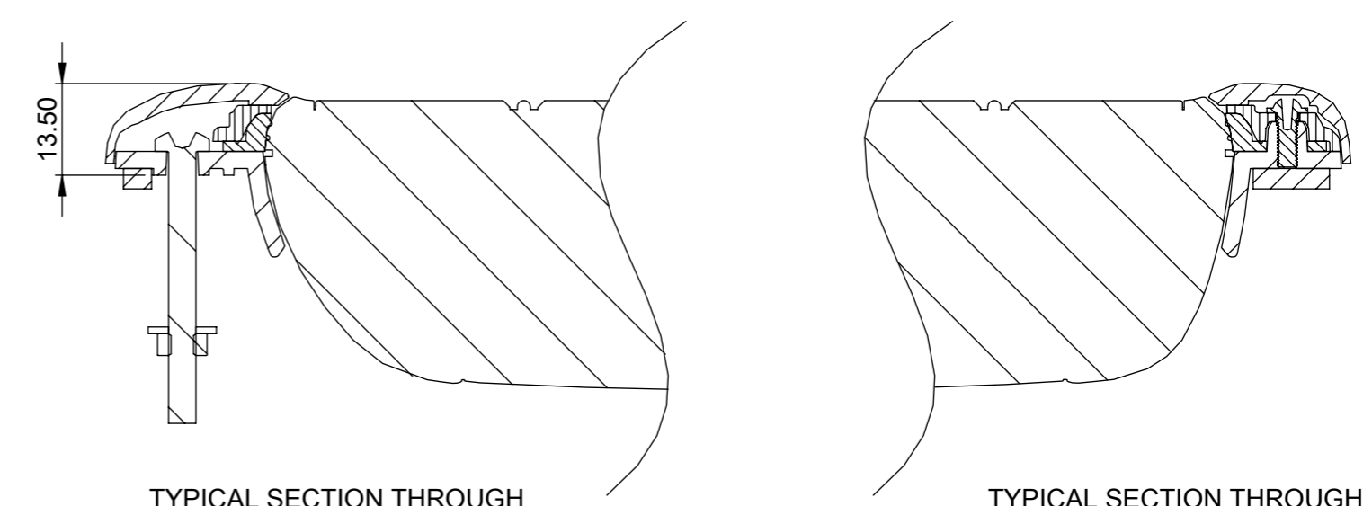
SECTION A-A SCALE 1 : 1
